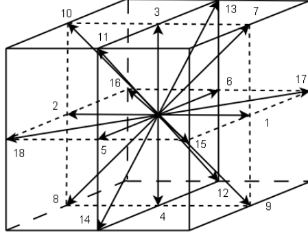
Fig. 1: D3Q19 model
